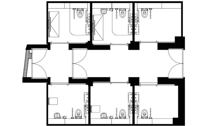
3F北東デッキ バリアフリートイレ図面
