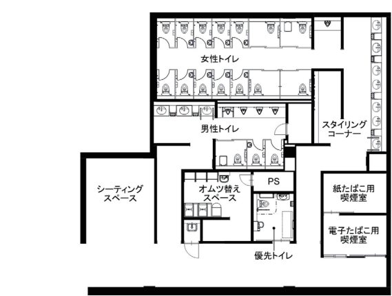
アウトレットゾーン1F トイレ図面
